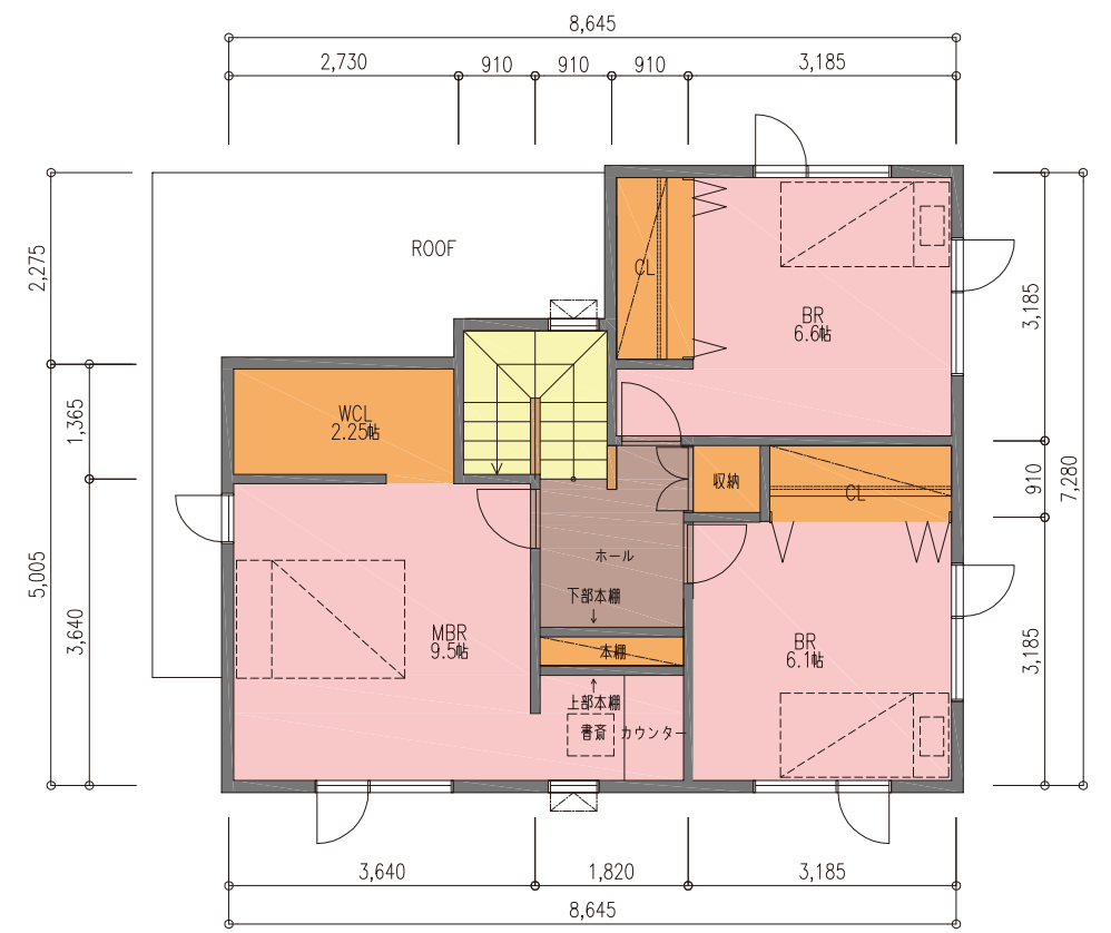
2階平面図
